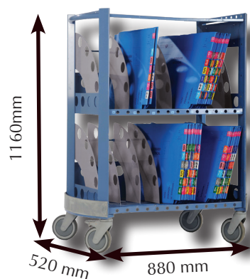
DROM standard 2 niveaux pour dossiers radio (2x70 cm), 12 intercalaires mobiles.
